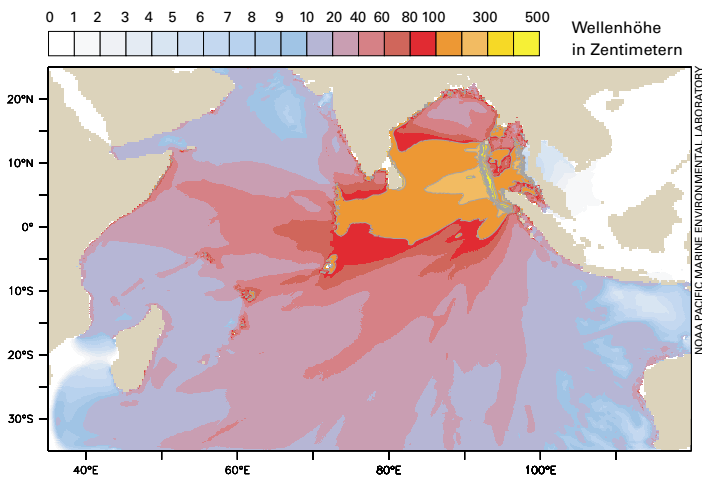
▲ Auf dem freien Meer war die Tsunamiwelle maximal vier Meter hoch, an der Küste Sumatras erreichte sie dagegen mehr als zehn und selbst am Horn von Afrika noch vier Meter Höhe.
