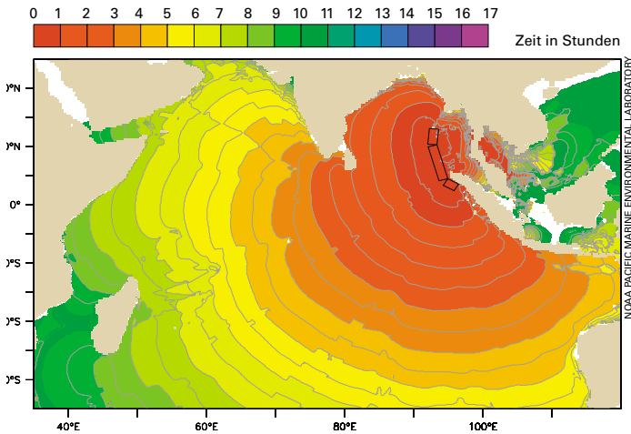
▲ Bei einer Geschwindigkeit von etwa 700 Kilometer pro Stunde erreichte die Tsunamiwelle nach etwa zwanzig Minuten Sumatra, nach drei Stunden Indien und nach acht Stunden Somalia am Horn von Afrika.
