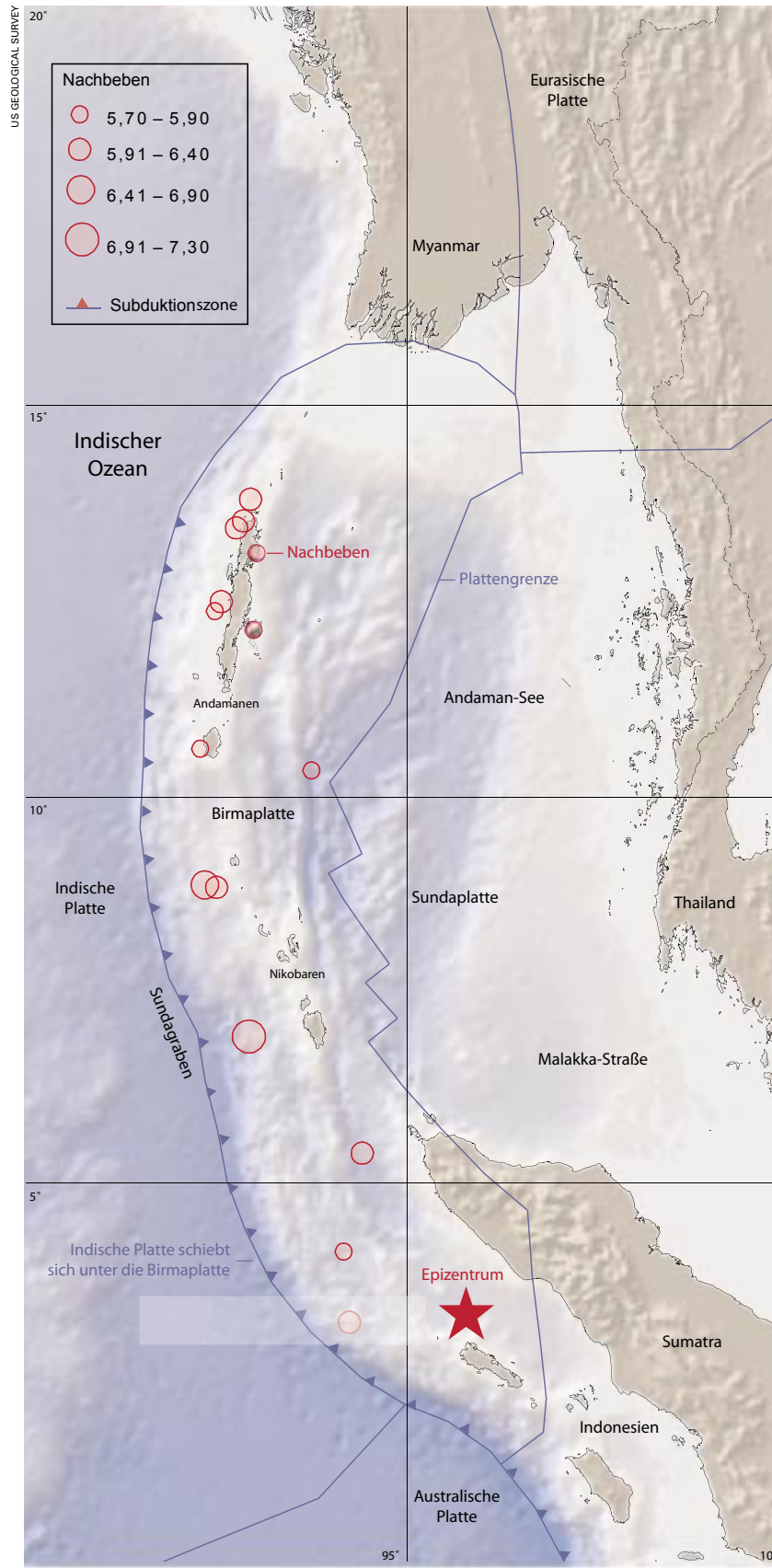
▲ Der verheerende Erdstoß am 26. Dezember (Stern) und die Nachbeben ereigneten sich an einem Abschnitt des Sundagraben, an dem die Indische Platte unter die Birma-Platte abtaucht.
