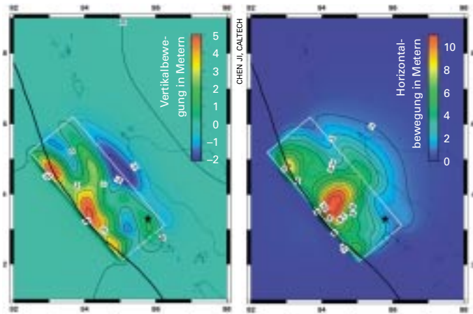
▲ Nach Modellrechnungen wurde der Meeresboden an dem Abschnitt der Plattengrenze, der an das Epizentrum des Bebens grenzt, um bis zu fünf Meter gehoben (links) und elf Meter horizontal versetzt (rechts).
