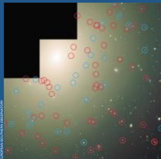
NGC 4365 enthält alte und mittelalte Kugelsternhaufen
